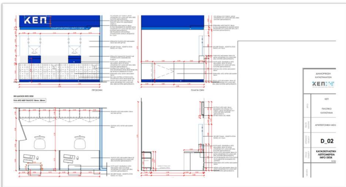
Τυπικό Σχέδιο D_02
