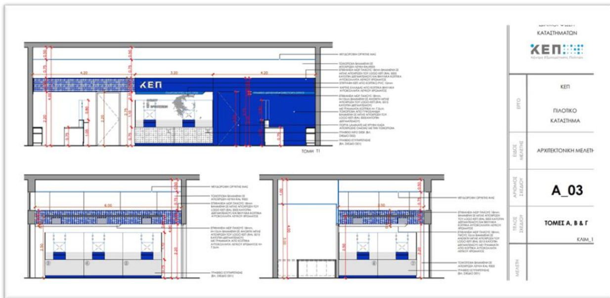
Τυπικό Σχέδιο A_03
