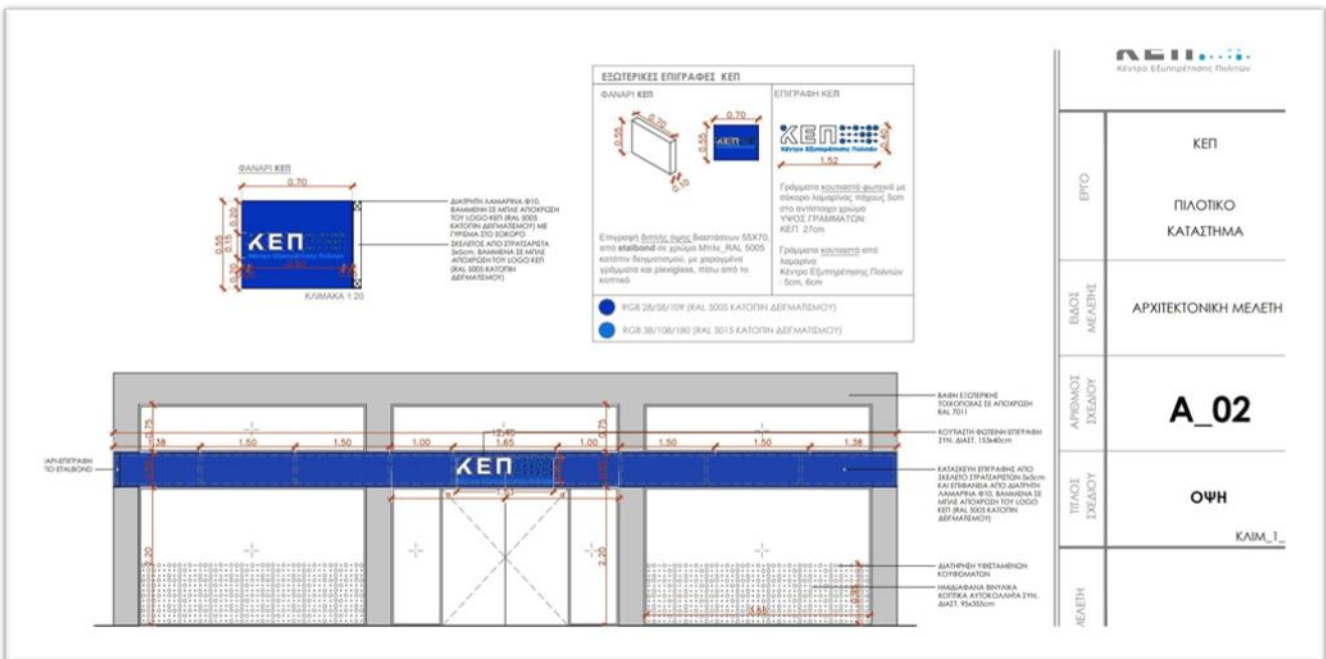
Τυπικό Σχέδιο A_02
