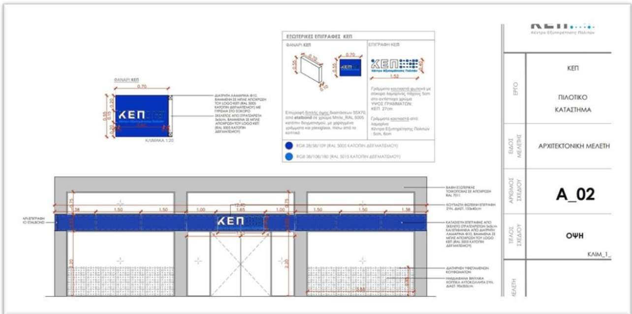
Τυπικό Σχέδιο A_02
